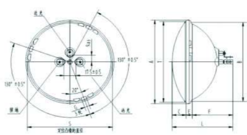
QF178外形图
