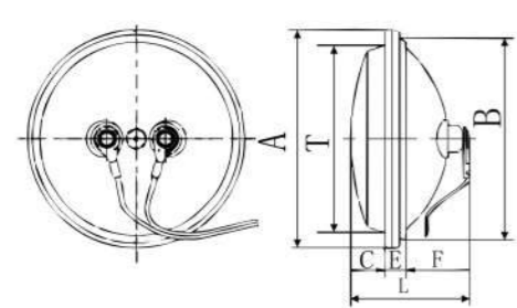
SF87外形图
