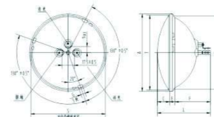
HIDSF142外形图
