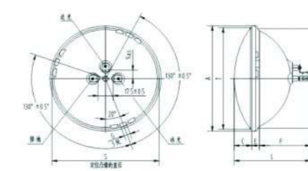
HSF178外形图
