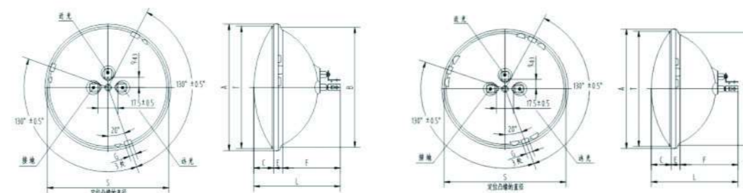
SF142外形图
