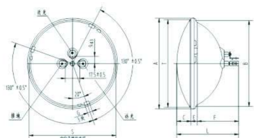
QF142外形图
