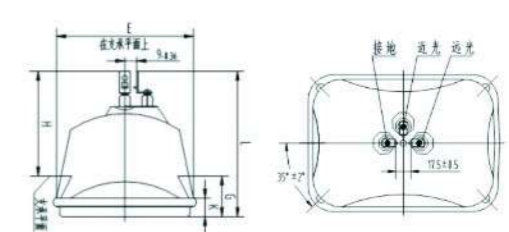
HIDSF165外形图
