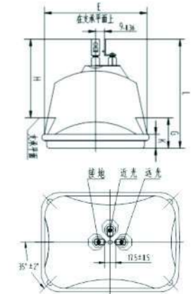
SF165外形图
