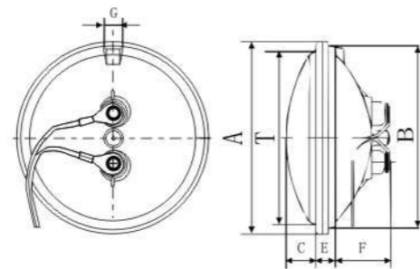
SF112外形图
