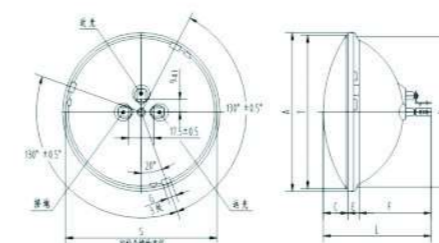
HSF142外形图
