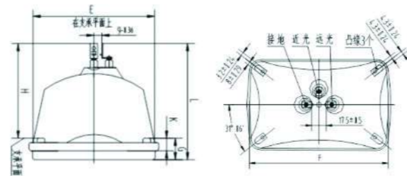
HSF190外形图
