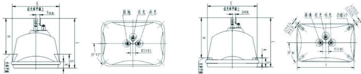
QF165外形图
