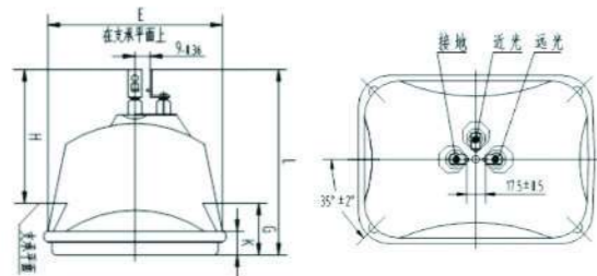
HSF165外形图
